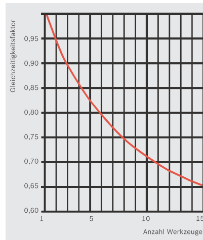
Abb. 3 Gleichzeitigkeitsfaktor
