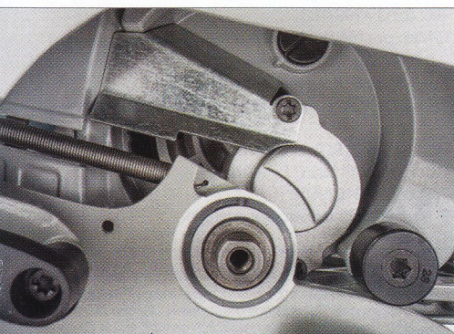
Gut 10 mm hat Bosch die Sägeblattaufnahme nach unten versetzt. Damit sind Schnitttiefen möglich, die sonst deutlich größere Blattdurchmesser erfordern
