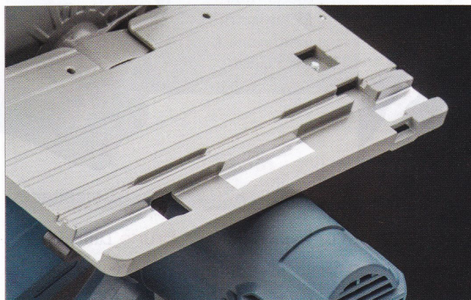
Die sauber gefräste Nut für die Führungsschiene passt auch auf Schienen anderer Hersteller
